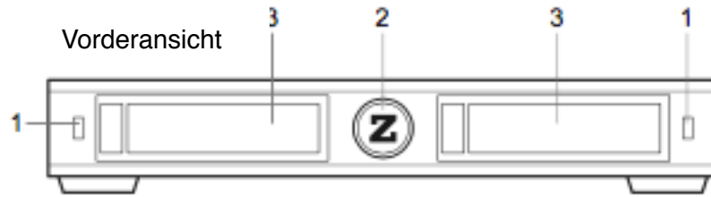
1. USB 2.0 Anschluss 2. LED Leuchte 3. Festplatteneinschub
